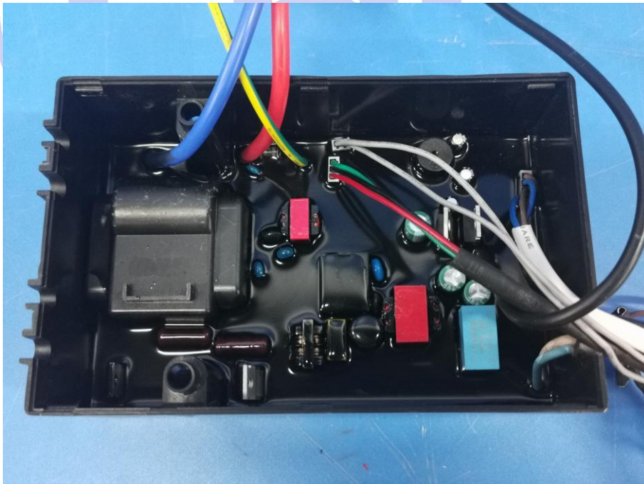
内部结构(控制器型号：DBD-B2, 点火器型号：DBD-A)
