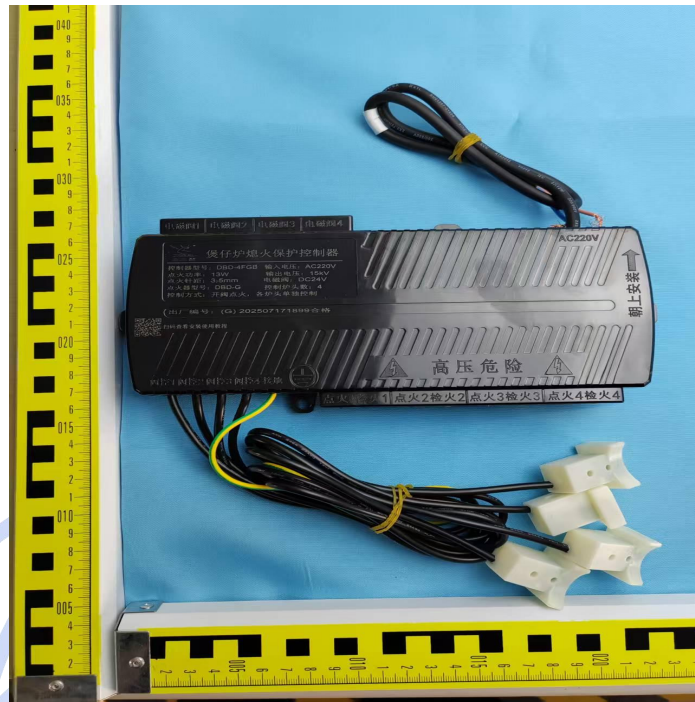
型号 DBD-4FGB 外观照片
