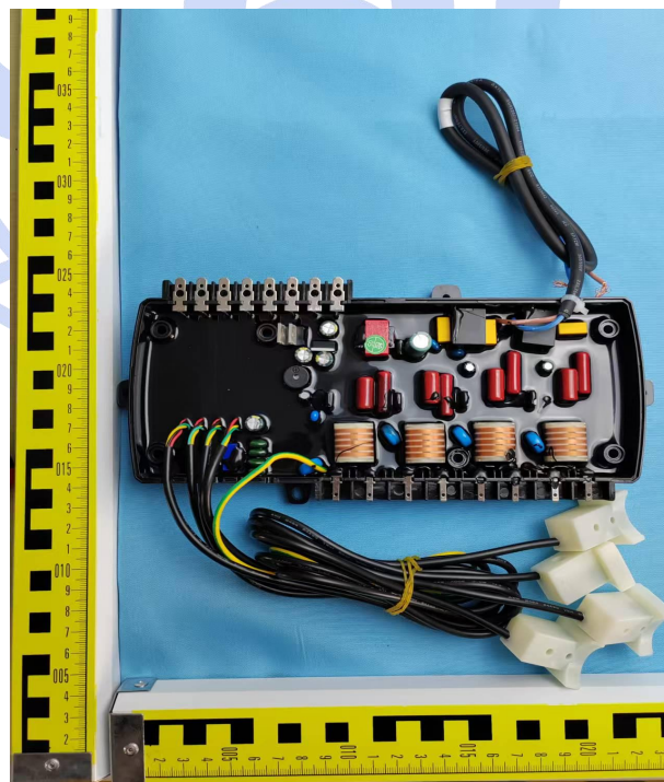
型号 DBD-4FGB 内部结构
